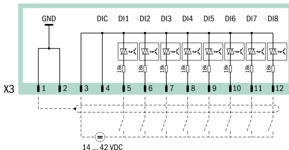
Steckverbinder X3 (Digitaleingänge)
