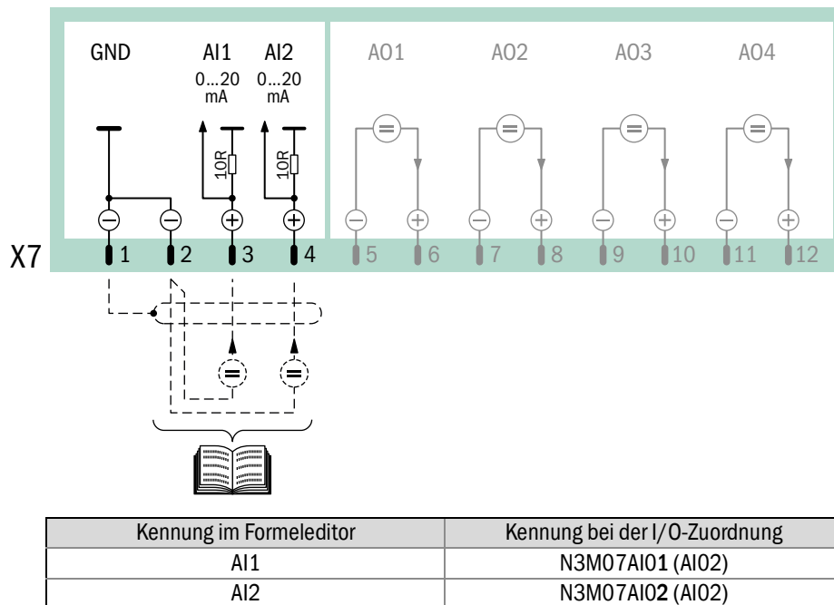
Bild 3 Steckverbinder X7 (Analogeingänge)
