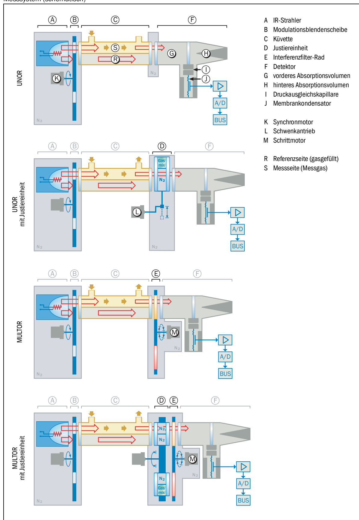
Messsystem (schematisch)
