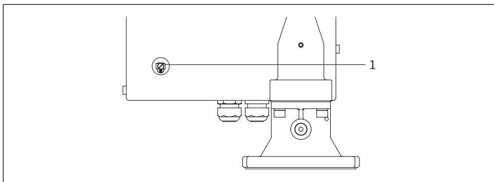
5 Potenzialausgleich anschließen
